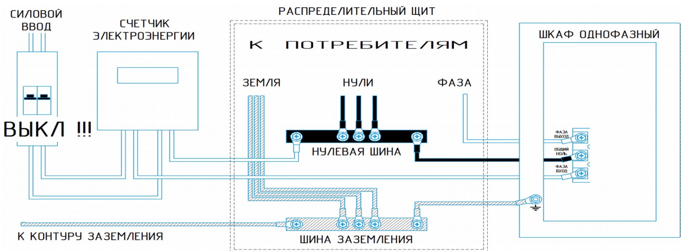
Рекомендованная схема подключения шкафа 1F TOP
